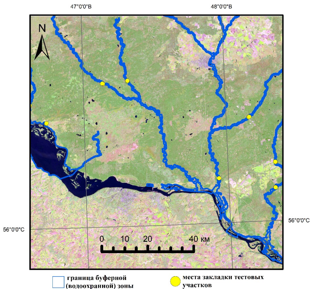
Рис. 1. Водоохранная зона на сцене T38VRH спутника Sentinel-2 на территорию Марийского Заволжья и распределение мест закладки тестовых участков
